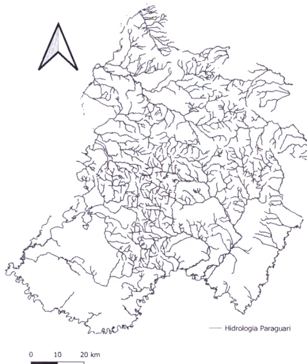
Figura 1. Mapa Hidrológico-Departamento de Paraguari
