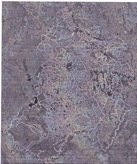
Figura 3. Puntos recorridos-Zona Arroyo Yukyry
